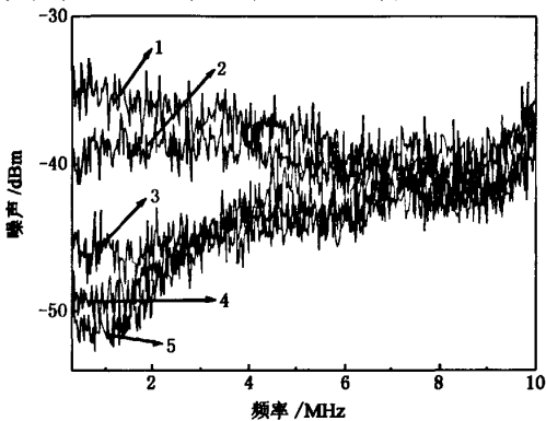
图 5 改变抽运激光器的功率在铷泡后测得的强度噪声谱(曲线 1—5 分别为 220,160,120,80,20 mW)
