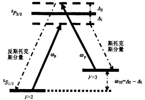
图 2 ^{85}\text{Rb} 原子的跃迁能级图
