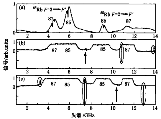
图 3 (a) Rb 原子 D_2 线的饱和吸收光谱, (b) 和 (c) 分别是耦合光在不同失谐位置时得到的拉曼增益峰和吸收峰
